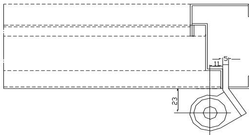
4 Нижний торец дверной коробки
