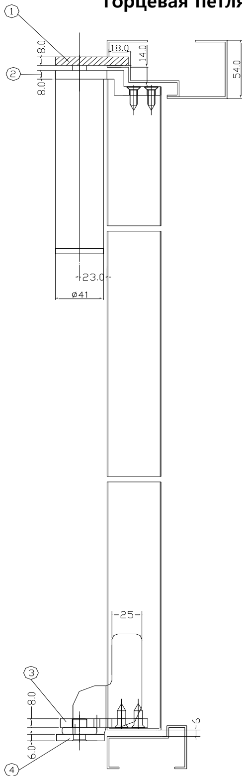
1 Верхний торец дверной коробки
