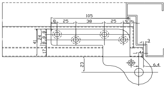
4 Нижний торец дверной коробки
